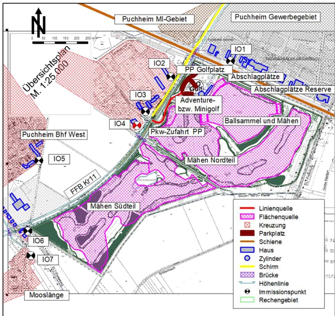
Abbildung 4. Übersichtslageplan Schallquellen und Immissionsorte.
